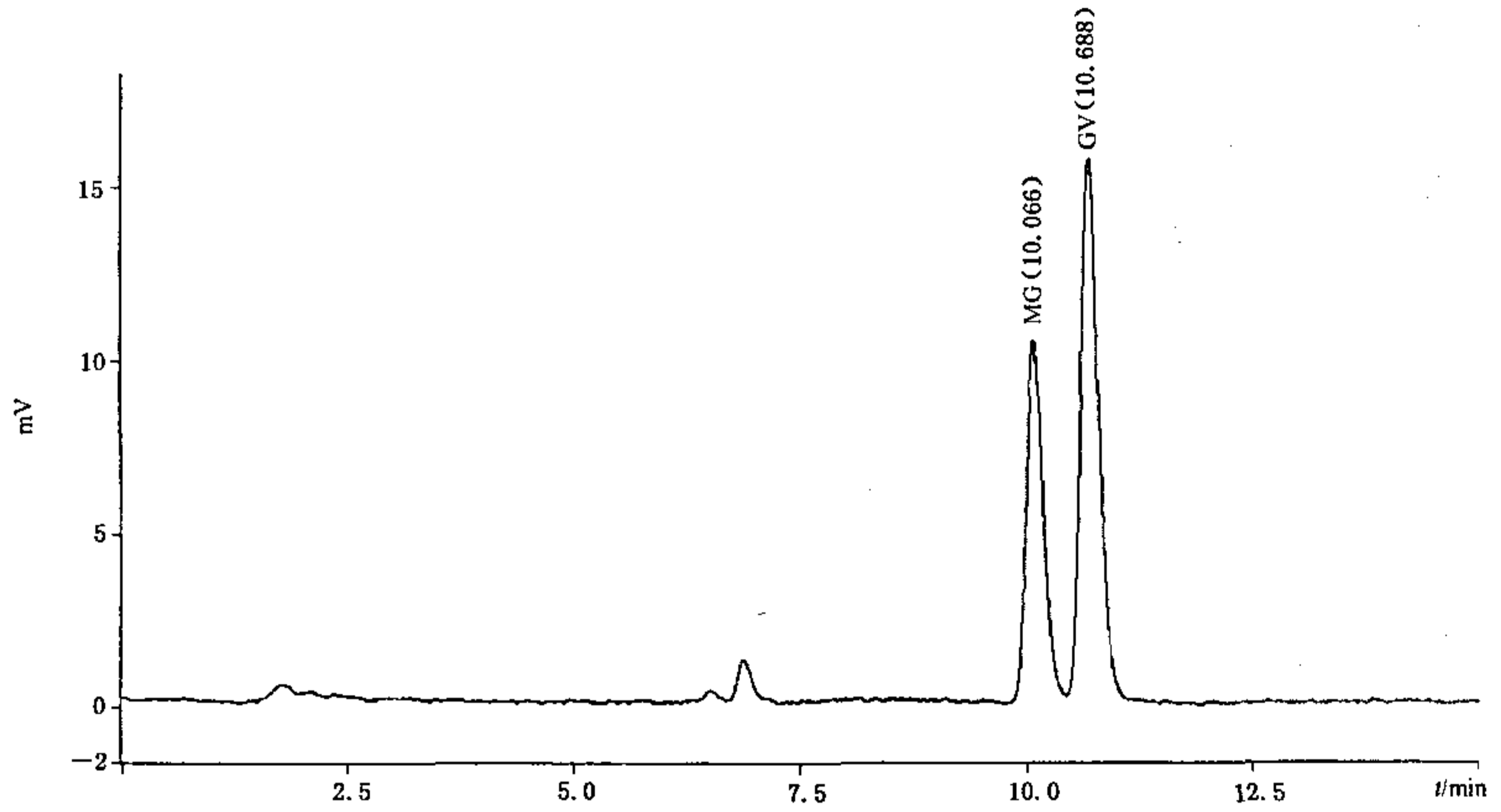
图 A.1 浓度为 0.01 \mu\text{g}/\text{mL} 孔雀石绿(MG)和结晶紫(GV)混合标准的液相色谱图
