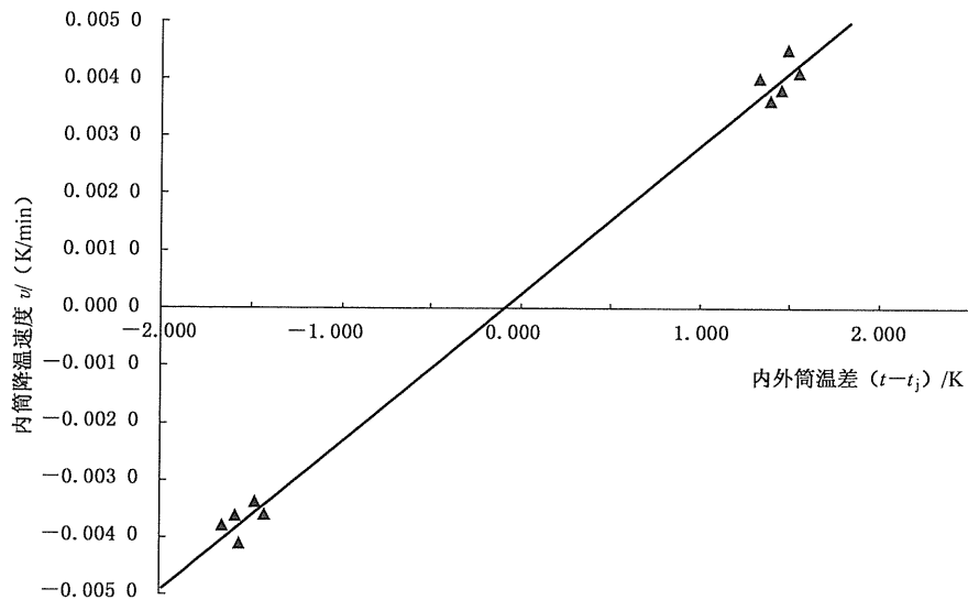
图1 v \sim (t-t_j) 关系曲线
