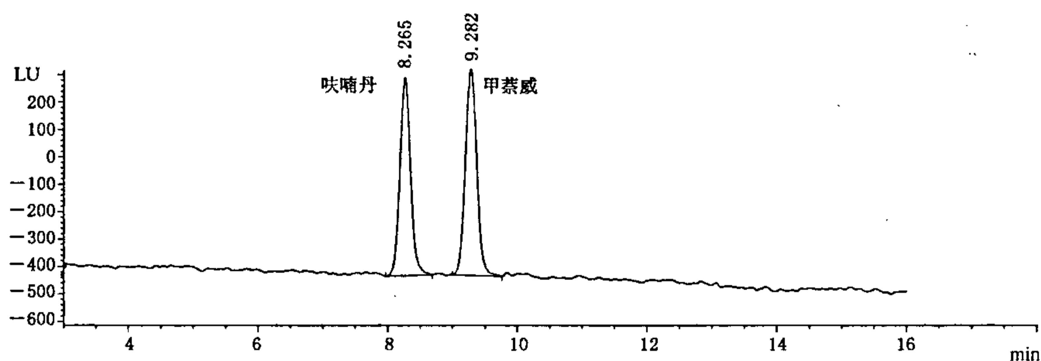
图 10 呋喃丹和甲萘威的标准色谱图
