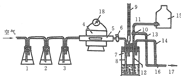
1—盛有 50 g/L 硫酸铜溶液的洗气瓶; 2—盛有 50 g/L 高锰酸钾溶液的洗气瓶; 3—盛有浓硫酸的洗气瓶; 4—管式电炉; 5—燃烧管和燃烧舟; 6—三通活塞; 7—吸收瓶; 8—圆形玻璃漏斗; 9—滴定管; 10—三通 活塞; 11、13、14—橡皮管; 12—玻璃管; 15—盛吸收液的下口瓶; 16、17—玻璃抽气管(或真空泵)和废液 排出口; 18—铂铑温度计
