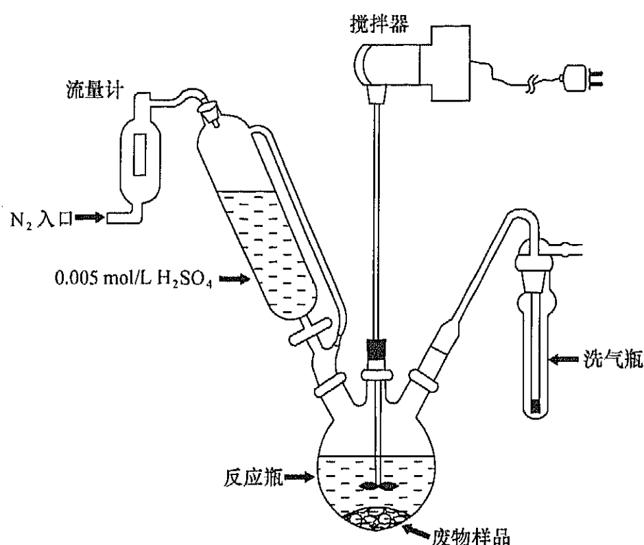
图 A.1 测定废物中氰化物或硫化物释放的实验装置
