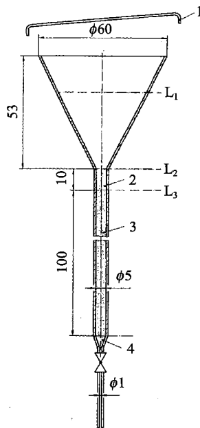
1—还原柱盖子; 2—填充的棉花; 3—处理后的镉粉 (颗粒直径为 0.3~0.8 mm); 4—填充的棉花
